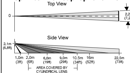
Рис. 6 Диаграмма направленности вертикальной барьерной линзы
