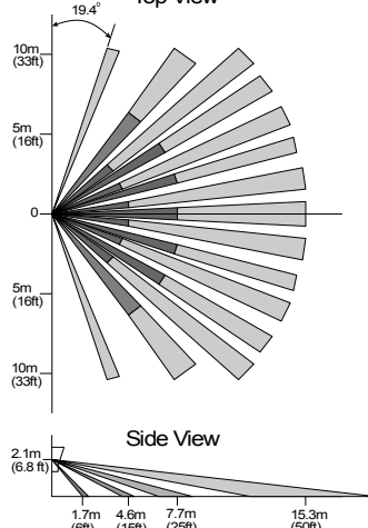
РИС. 4 ДИАГРАММА НАПРАВЛЕННОСТИ ШИРОКОУГОЛЬНОЙ ЛИНЗЫ Top View
