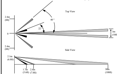
Рис. 6 Диаграмма направленности вертикальной барьерной линзы
